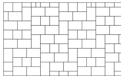
Muster 10 Format 20 x 20 cm, Bedarf ca. je m 2 7,5 Stück Format 30 x 20 cm, Bedarf ca. je m 2 11,7 Stück Randabschluss Format 20 x 10 cm, Bedarf ca. 2,5 Stück je lfd. M. Format 10 x 10 cm, Bedarf ca. 1,0 Stück je lfd. M.
