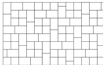
Muster 11 Format 20 x 20 cm, Bedarf ca. je m 2 10,1 Stück Format 30 x 20 cm, Bedarf ca. je m 2 9,9 Stück Randabschluss Format 20 x 10 cm, Bedarf ca. 0,5 Stück je lfd. M.
