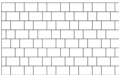
Muster 4 Format 30 x 20 cm, Bedarf ca. je m 2 10 Stück Format 20 x 20 cm, Bedarf ca. je m 2 10 Stück Randabschluss Format 20 x 10 cm, Bedarf ca. 2 Stück je lfd. M.
