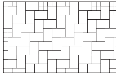
Muster 8 Format 30 x 20 cm, Bedarf ca. je m 2 16,7 Stück Randabschluss Format 10 x 10 cm, Bedarf ca. 9 Stück je lfd. M.
