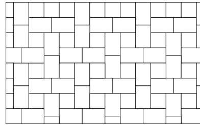
Muster 9 Format 30 x 20 cm, Bedarf ca. je m 2 12 Stück Format 20 x 20 cm, Bedarf ca. je m 2 7 Stück Randabschluss Format 20 x 10 cm, Bedarf ca. 4 Stück je lfd. M. Format 20 x 20 cm, Bedarf ca. 2 Stück je lfd. M.
