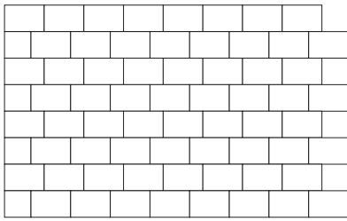
Muster 1 Format 30 x 20 cm, Bedarf ca. je m 2 16,7 Stück Randabschluss Format 20 x 20 cm, Bedarf ca. 3 Stück je lfd. M.
