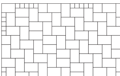
Muster 7 Format 30 x 20 cm, Bedarf ca. je m 2 16,7 Stück Randabschluss Format 10 x 10 cm, Bedarf ca. 5 Stück je lfd. M. Format 20 x 20 cm, Bedarf ca. 1 Stück je lfd. M.
