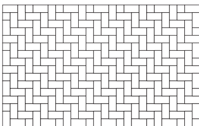
Muster 6 Format 20 x 10 cm, Bedarf ca. je m 2 50 Stück Randabschluss Format 10 x 10 cm, Bedarf ca. 2,5 Stück je lfd. M.
