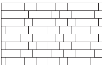
Muster 5 Format 30 x 20 cm, Bedarf ca. je m 2 : 13,6 Stück Format 20 x 20 cm, Bedarf ca. je m 2 4,6 Stück
